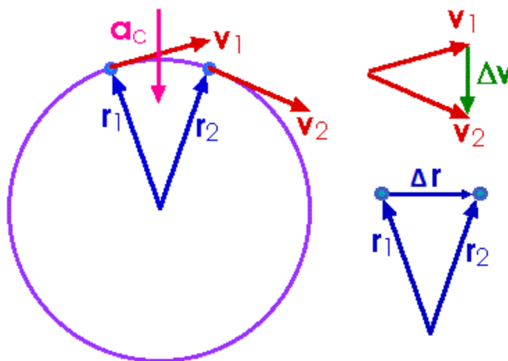
Figur 3.8: Utledning av sentripetalakselerasjon
