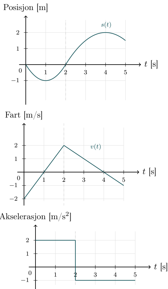
Figur 3.4: Posisjon, fart og akselerasjon ved varierende akselerasjon ( s_0 = 0 , v_0 = -2 \text{ m/s} ; a_1 = 2 \text{ m/s}^2 for t \in [0, 2 \text{ s}] og a_2 = -1 \text{ m/s}^2 for t \in [2, 5 \text{ s}] ).
