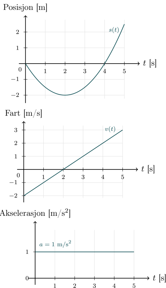
Figur 3.3: Posisjon, fart og akselerasjon ved konstant akselerasjon ( s_0 = 0 , v_0 = -2 \text{ m/s} , a = 1 \text{ m/s}^2 ).
