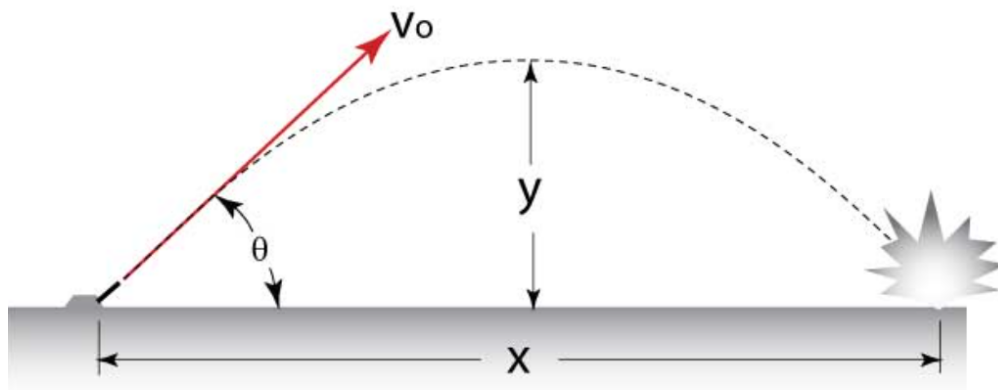
Figur 3.5: Prosjektilbevegelse
